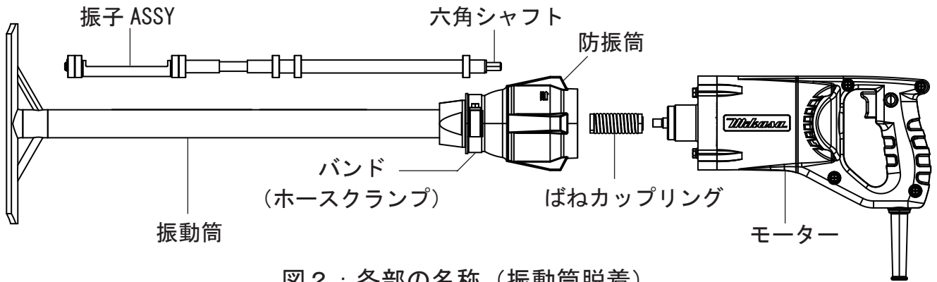
図 2 : 各部の名称 (振動筒脱着)
