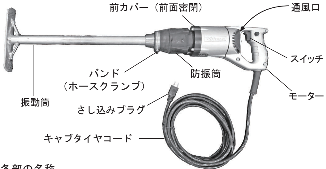
図 1 : 各部の名称
