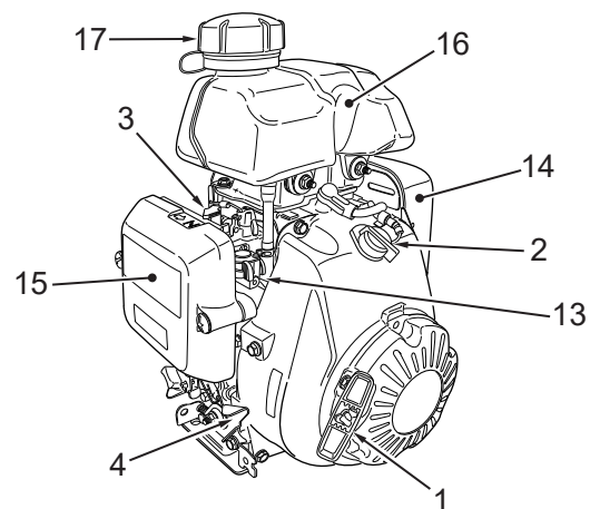
GX100型エンジン
