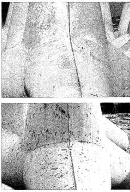
上はテトラポット用バイブレーターを使ったもの、下は通常のバイブレーターによる製品
