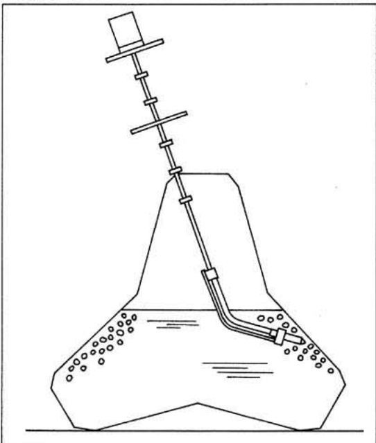
テトラポット用バイブレーターの使用概念図
