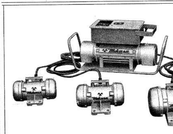
(左よりFM-400型・750型・1200型、後方は周波数変換器)
