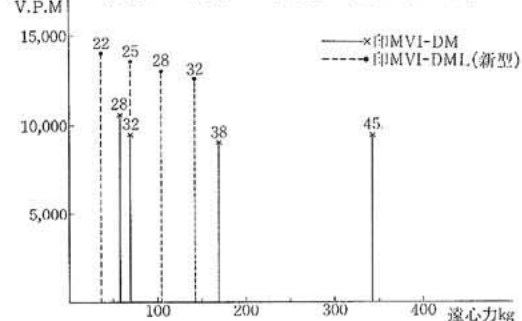
新製品と現製品の振動数と遠心力の比較
