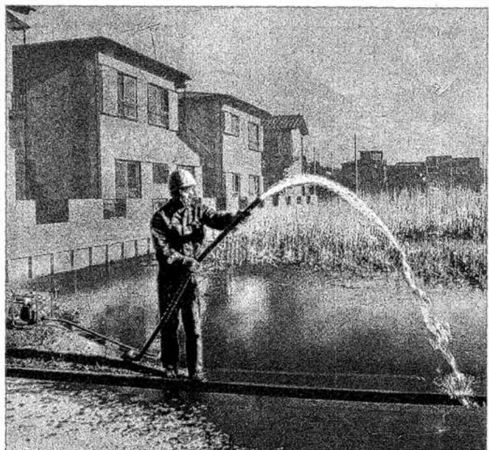
(排水作業中の MVP-MN 型ミニ・フレキシブル水中ポンプ)
