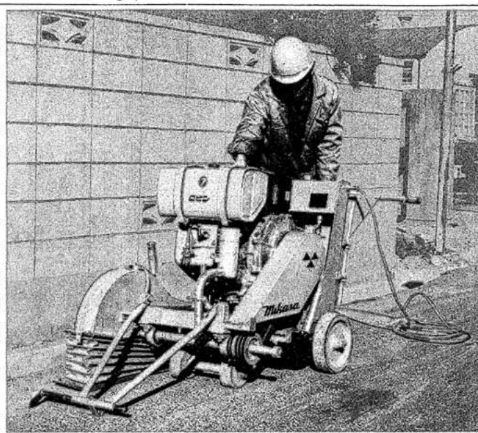
(3型コンクリートカッターに取付けられた防音カバーをセットしての作業状況)
