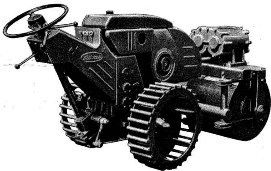
スパイク車輪を取付けた三笠MRV-10型インパクトローラー（小型振動ローラー）
