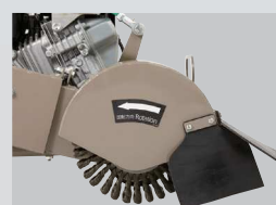
③ ブレードカバー・ワイヤーブレード取付
