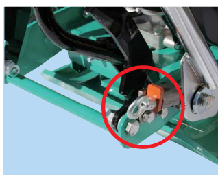
ハンドル固定用ノブ(ロック装置) ● 運搬時はロック ● 転圧作業時はロックを解除
