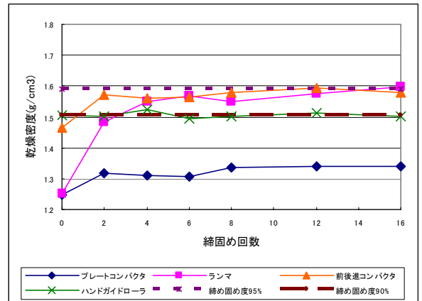
図-4 乾燥密度 (深さ 200~300mm)
