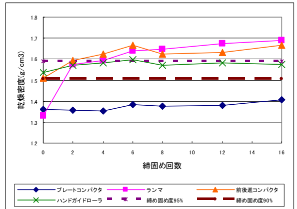
図-3 乾燥密度 (深さ 100~200mm)
