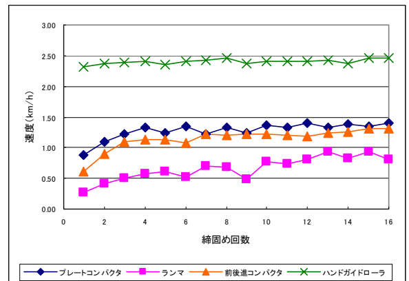
図-5 機械走行速度
