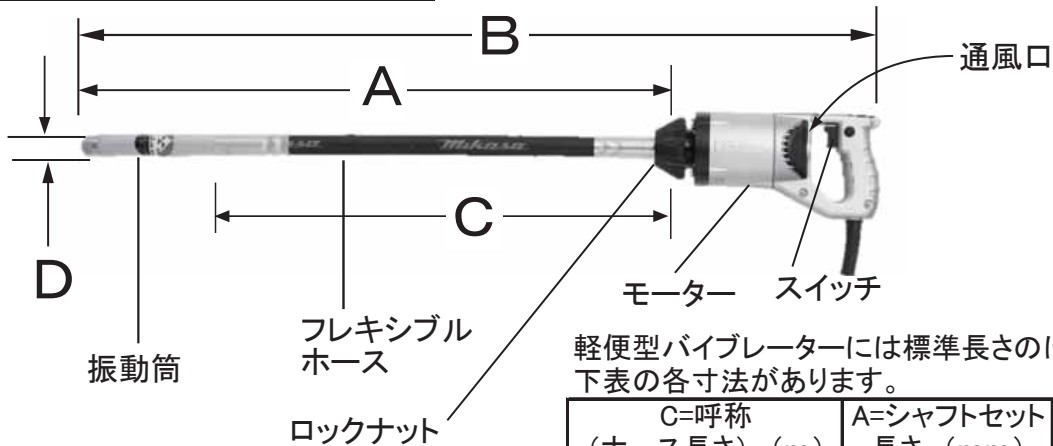
図1：各部の名称
